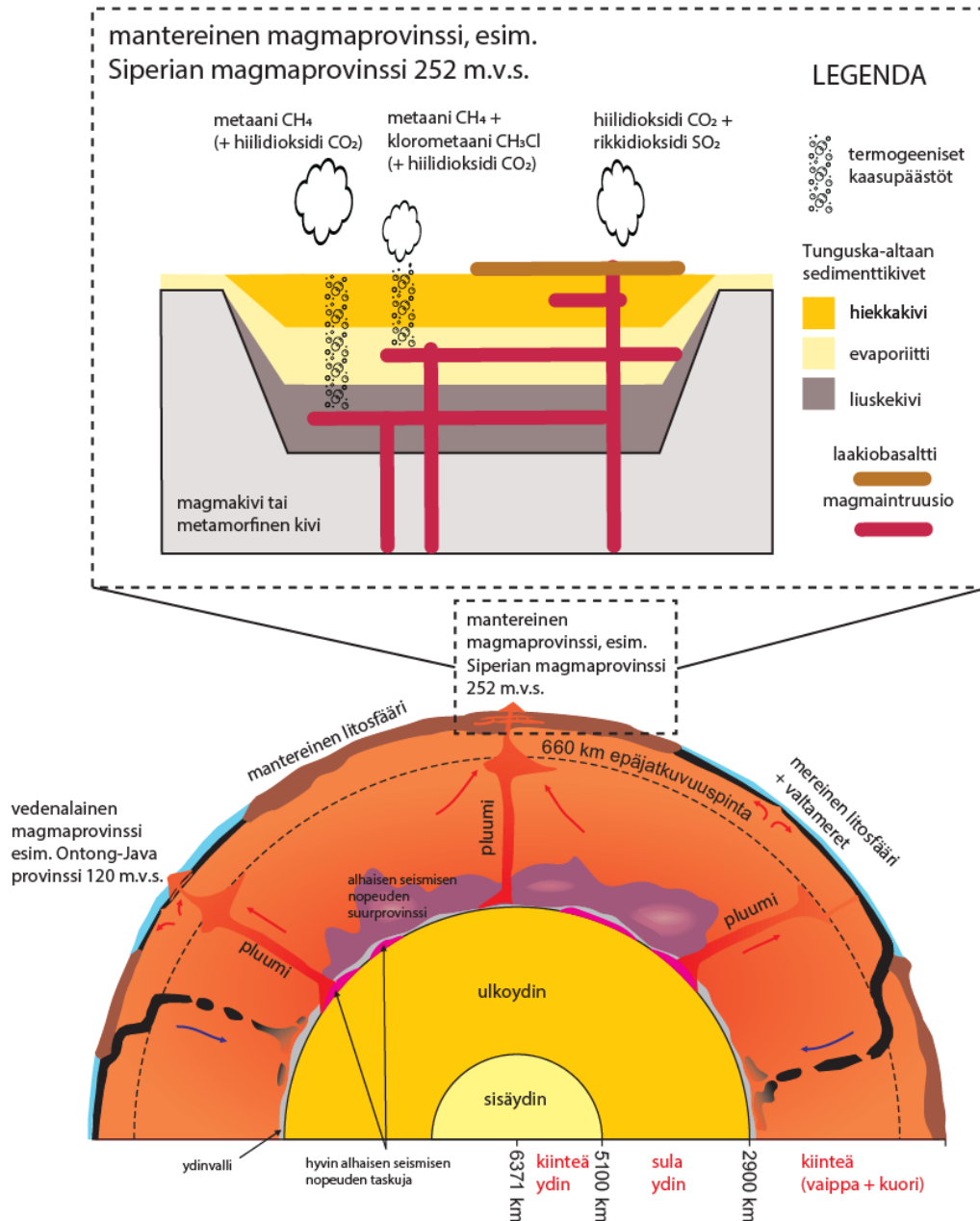
Kuva 3.1. Maan rakenne (alempi), jossa näkyy ydin, vaippa, mantereinen kuori sekä mereinen kuori. Kivisulan pluumit nousevat pystysuunnassa pintaa kohti ja voivat aiheuttaa nk. suuria magmaprovinssseja (ylempi). Kun suuri magmaprovinssi esiintyy mantereisessa ympäristössä, kaasuja vapautuu ilmakehään suoraan magmasta, mutta myös sedimenttikivistä, joiden kautta magma kulkee matkallaan pintaan. Huomaa, että kaasun koostumus riippuu kivityypistä, josta päästö on peräisin. Lyhenne m.v.s. tarkoittaa miljoonaa vuotta sitten. Kuva on muokattu Suomen muinaiset tulivuoret – blogin (Jussi Heinonen, Elina Lehtonen, 2022) ja Svensen et al. 2023 artikkelin mukaan.
