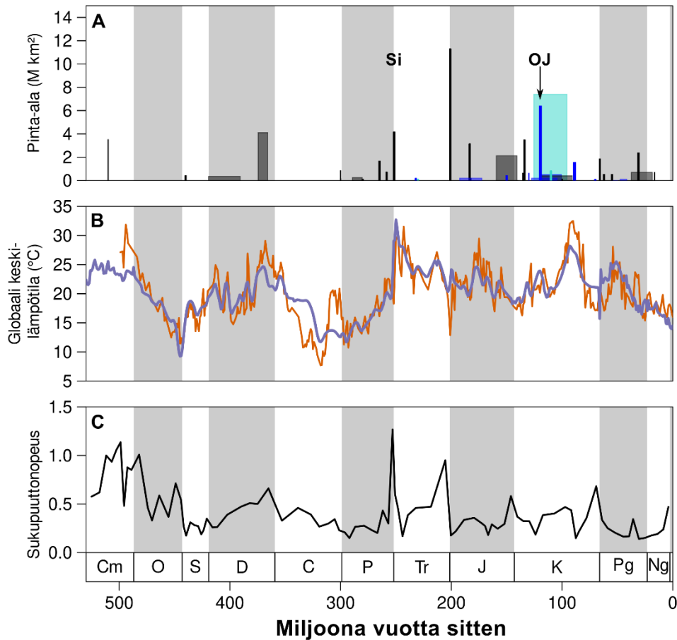
Kuva 3.4 Suurten magmaprovinssien yhteys ilmastomuutokseen ja sukupuuttoihin. A: Suuren magmaprovinssin purkausalueen pinta-ala. Pylvään paksuus kuvaa purkauksen ajallista kestoa. Pylvään väri puolestaan kuvaa purkausympäristöä. Musta/tummanharmaa pylväs: purkaus tapahtui mantereella; sininen pylväs: purkaus tapahtui merellisen kuoren päälle; turkoosi pylväs: purkaus tapahtui osin mantereella osin merellisen kuoren päälle. Kuvaan on esimerkkeinä merkitty myös Siperian (Si) ja Ontong-Javan (OJ) suuret magmaprovinssit (Ernst et al. 2021). B: Kaksi eri menetelmiin perustuvaa globaalin keskilämpötilan rekonstruktioita (Scotese et al. 2021; Shaviv et al. 2023). C: Sukupuuttoonopeus valtamerissä (Kocsis et al. 2019). Vaikka kuvaaja esittääkin sukupuuttoja meriekosysteemeissä, se kuvastaa sukupuuttojen ajankohtia ja voimakkuutta myös mantereilla.
