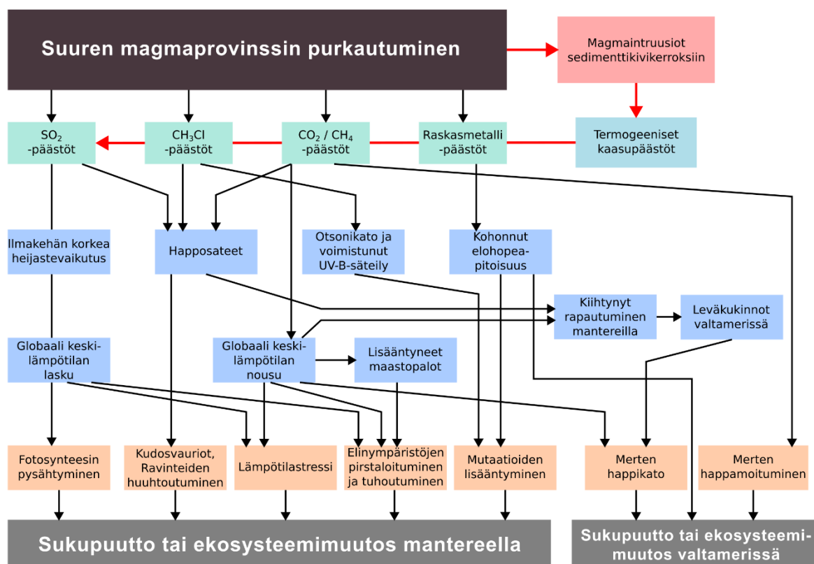
Kuva 3.3. Suuren magmaprovinssin purkautumisen ekosysteemivaikutuksia kuvaava vuokaavio (mukaillen Grasby & Bond, 2023, Galloway & Lindström 2023)
