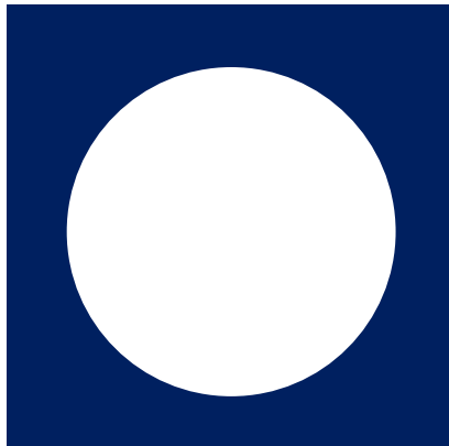
Täysikuu
