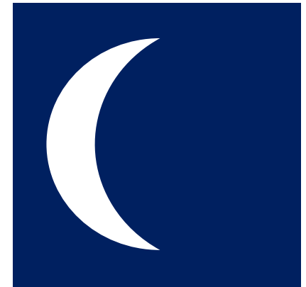
Pienenevä sirppi
