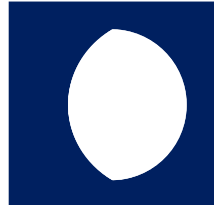
Kasvava kuperakuu
