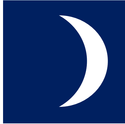
Kasvava sirppi
