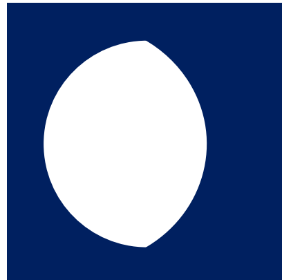
Pienenevä kuperakuu
