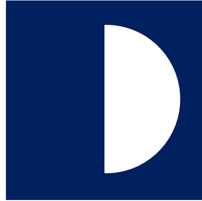
Kasvava puolikuu
