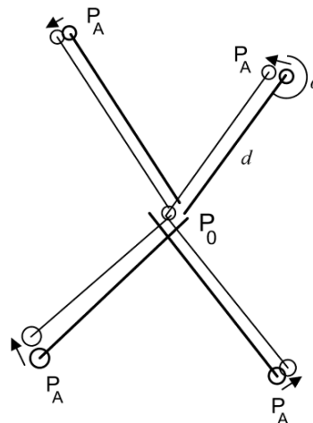
2.0c. Kohteen ( P_0 ) paikannus ilmakuva puiden ( P_A ) avulla, kun havaitaan pisteiden välisiä atsimuutteja ( \alpha ) ja/tai etäisyyksiä ( d ). Tasoituslaskennan seurauksena tuntematon piste "hakeutuu" paikkaan, jossa havaintojen (ilmakuva puiden P_A XY-koordinaatit, puiden väliset suunnat, puiden väliset etäisyydet) residuaalien poikkeamien neliösumma minimoituu. Myös ilmakuva puille sallitaan pieni "tasoittava" liike.
