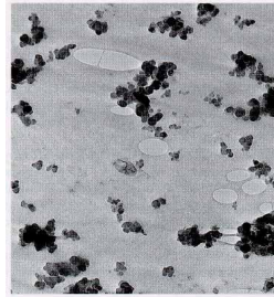
Gummi förstärkt med kolsvart, x80000. Hålena är luftbubblor
