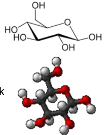
Strukturen av glukos [Wikipedia]
