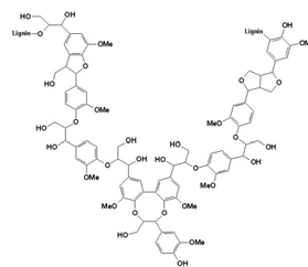
(del av lignin-polymer)
