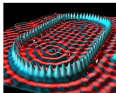
["Quantum corral", IBM]
