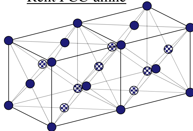
Rent FCC-ämne
