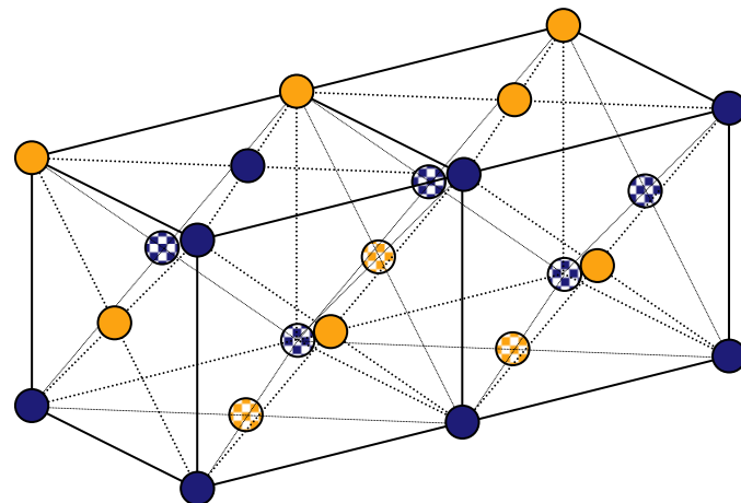
Oordnad FCC-legering
